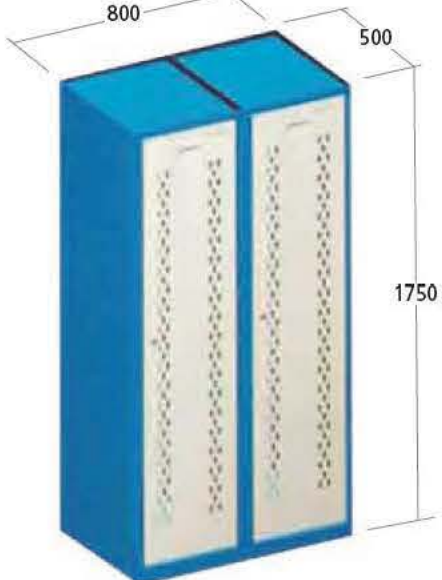
Vestiaire double 1 porte
